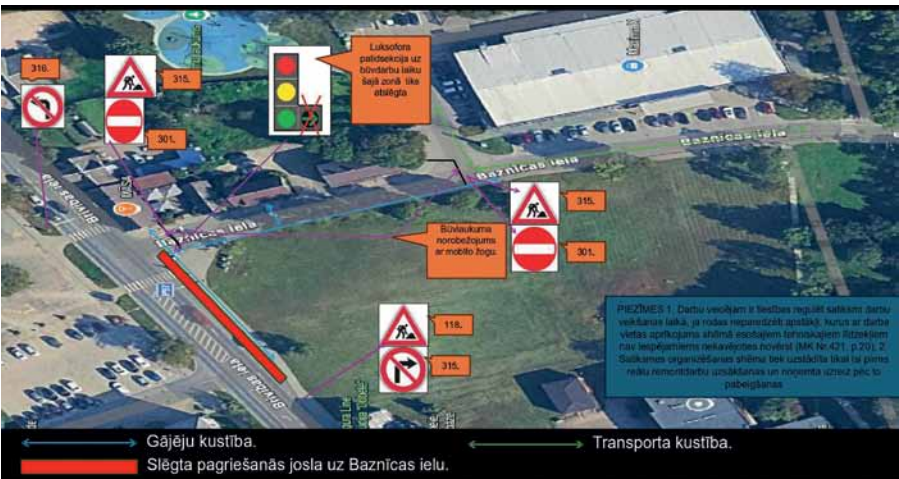
Satiksmes organizācijas shēma Baznīcas ielas vienkāršotās atjaunošanas būvdarbu laikā
