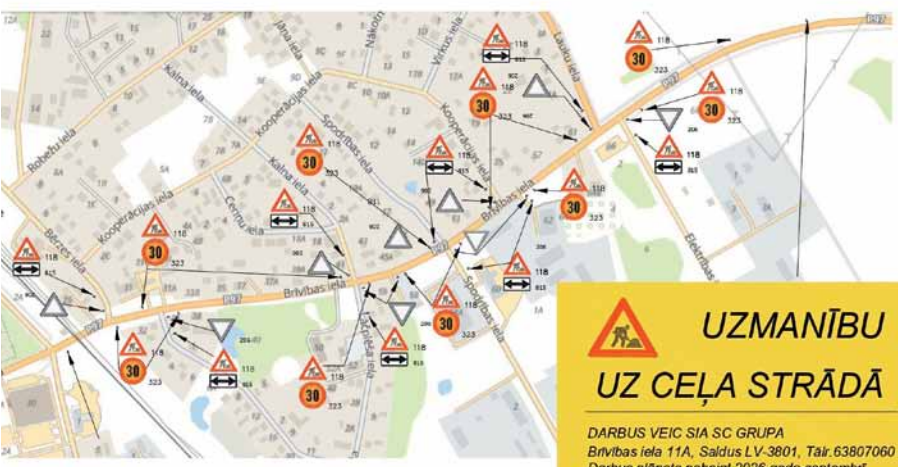
Satiksmes organizācijas shēma Brīvības ielas brauktuves dilumkārtas būvdarbu laikā
